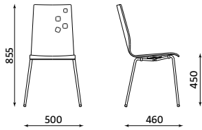
AMMI 4L
