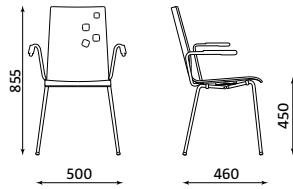
AMMI 4L-ARM
