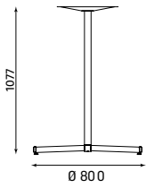
CRUZO LARGO 1100 Ø 800
